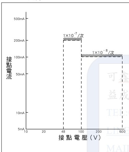
圖1. S(D)-T主接點
