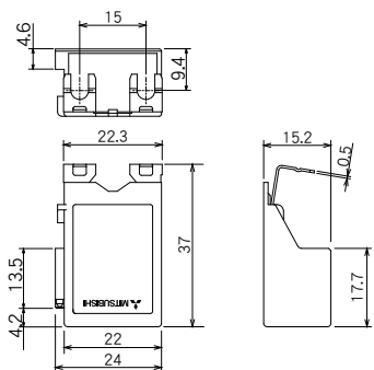
安裝後的電磁接觸器、電磁繼電器的外形尺寸不變。
