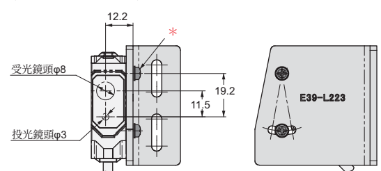
安裝感測器時的尺寸 (例：E3AS-HL500□)
