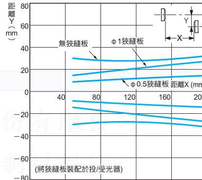
動作領域特性
