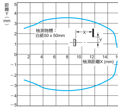
BGS反射型 E3T-FL1□型
