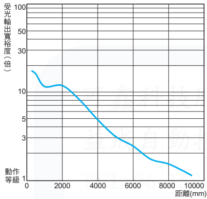
E3T-FT1□型
