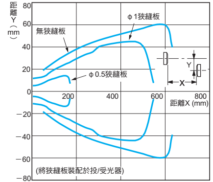
E3T-FT2□型 + E39-S64型
