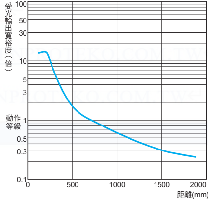
E3T-FT2□F型
