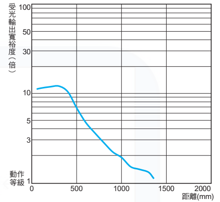
E3T-ST2□F型
