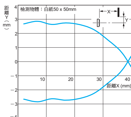
擴散反射型 E3T-FD1□(M)型
