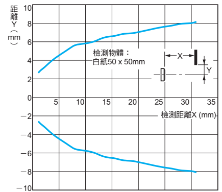
E3T-FL2□型
