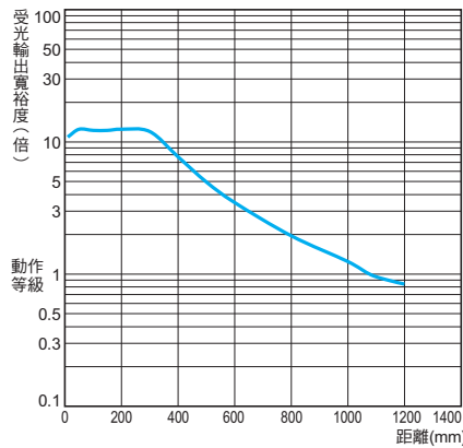
E3T-FT2□F型
