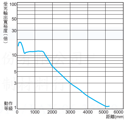
E3T-FT2□型
