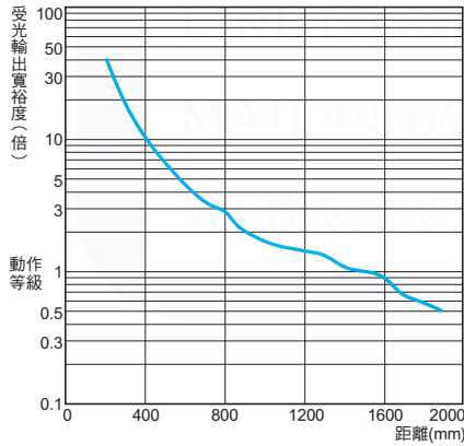
E3T-FT1□F型
