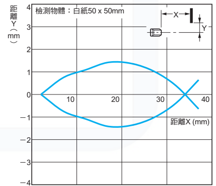
E3T-SL2□(M)型
