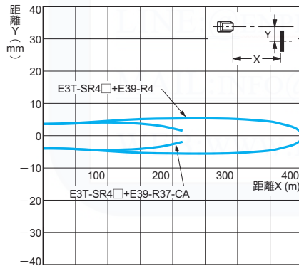
回歸反射型 E3T-SR4□型
