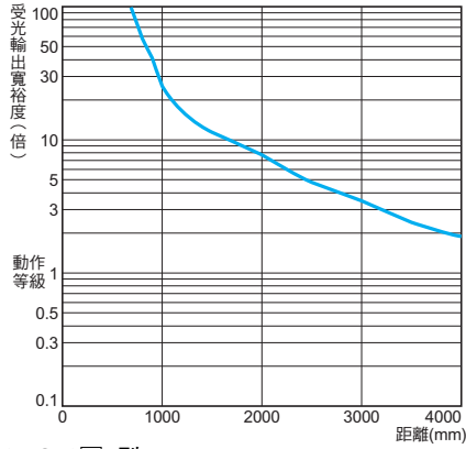
E3T-ST3□F型
