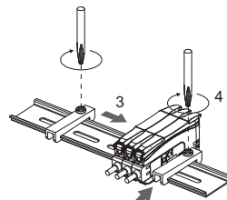
按住螺絲並同時鎖緊。
