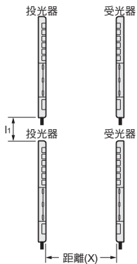
上下並排設置(垂直配置)
