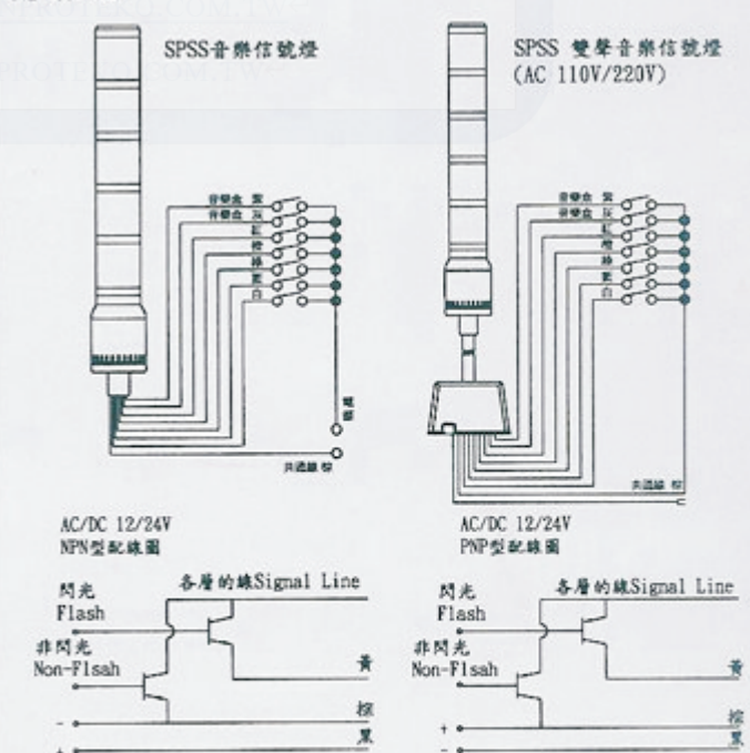
配線圖
