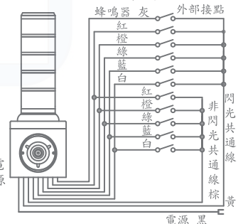
SCRS蜂鳴器閃光信號燈配線圖
