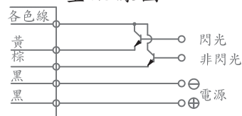
NPN型配線圖
