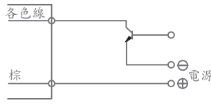
NPN型配線圖
