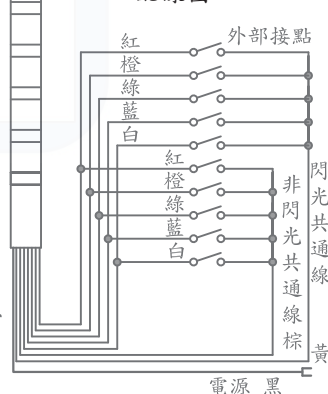
SCR閃光信號燈 配線圖
