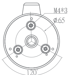
直付式開孔尺寸圖
