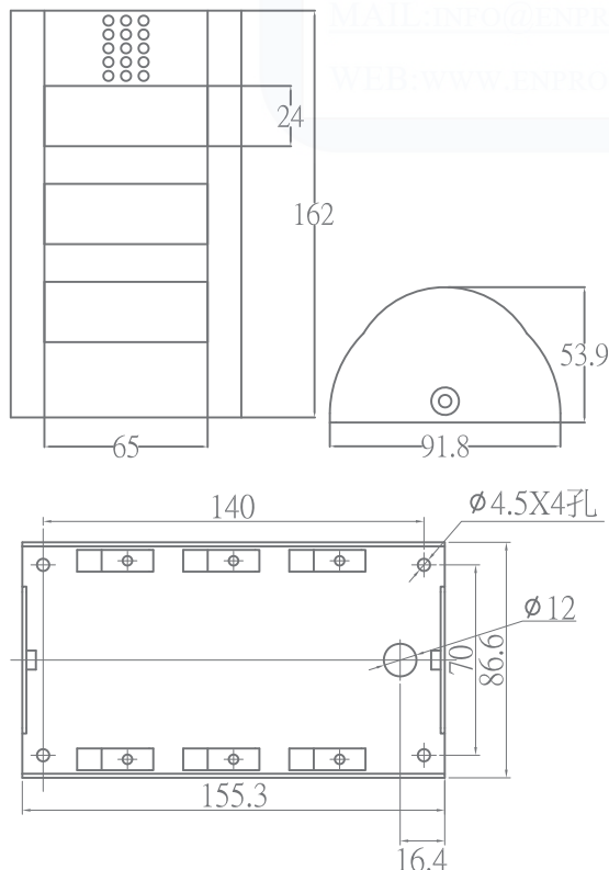
尺寸圖
