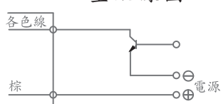
NPN型配線圖
