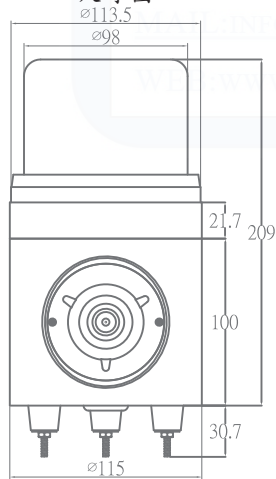
直付式開孔尺寸圖
