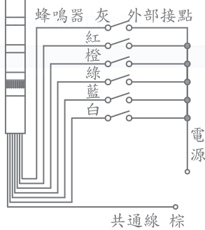
NPN型配線圖
