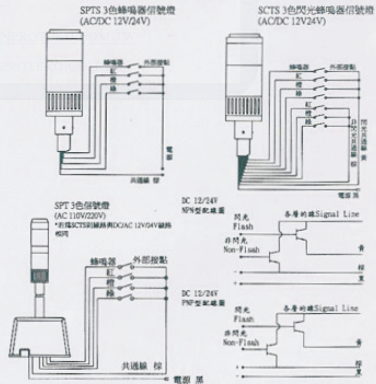
配線圖(此圖為32型若為35型則線路相同但外型不同)
