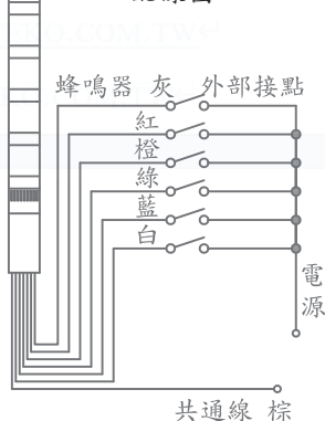
SPES蜂鳴器信號燈配線圖
