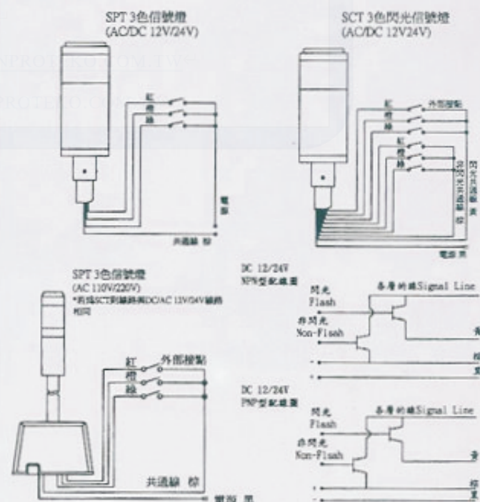
配線圖
