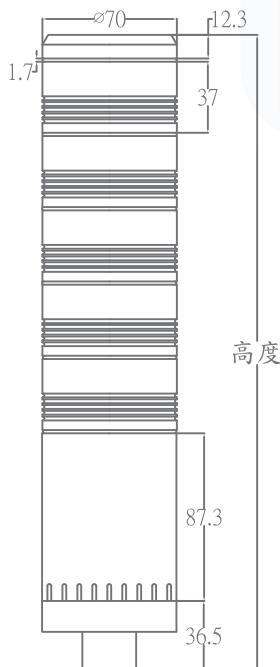
尺寸圖
