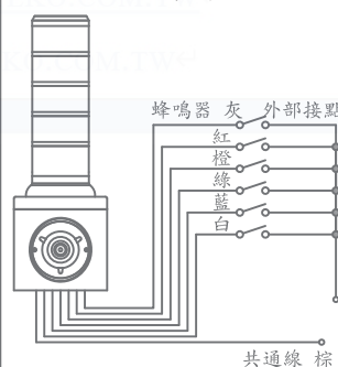
SPES蜂鳴器信號燈配線圖
