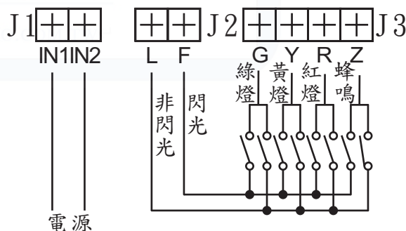
端子接線圖
