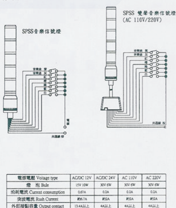
配線圖
