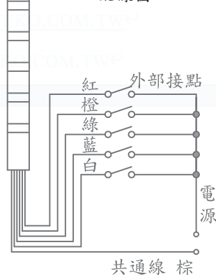
SPE信號燈 配線圖
