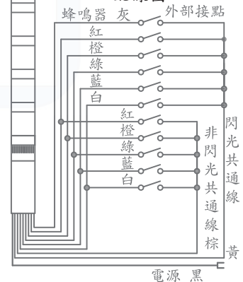
NPN型配線圖
