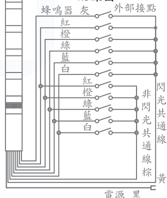
SCRS蜂鳴器閃光信號燈配線圖
