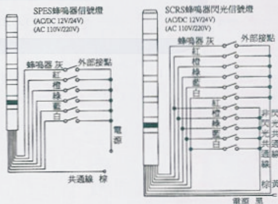
配線圖
