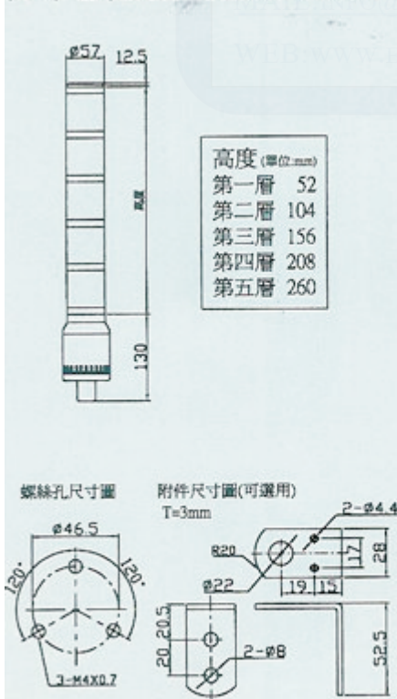
尺寸圖 (總高度=(層數×52)+130+12.5)
