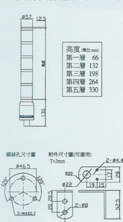
尺寸圖 (總高度=(層數X66)+130+12.5)
