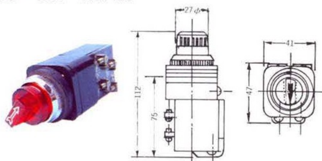
SIT-304 切替開關
